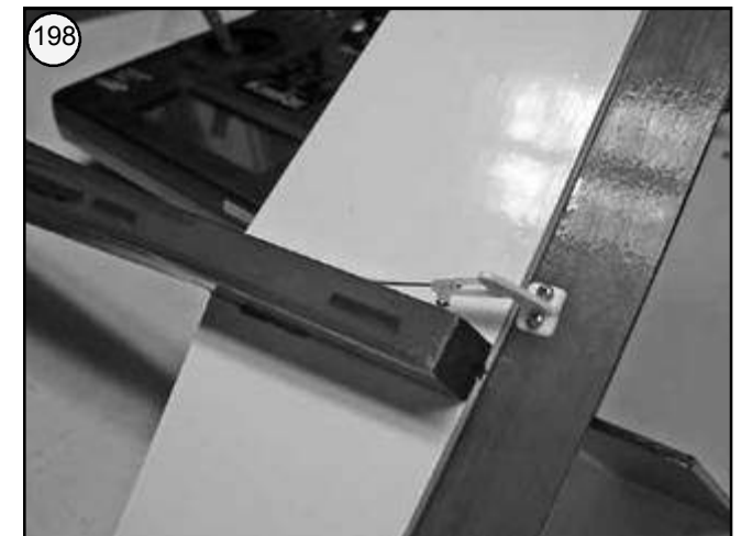
Bild 198 - Höhenruder in der gleichen Weise anlenken.
