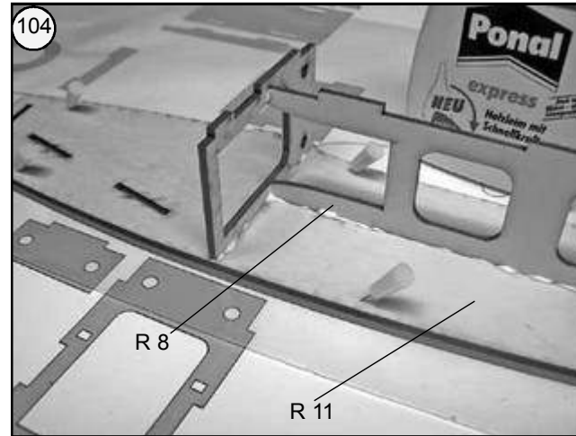
Bild 104 - Fertigen Innenrahmen auf die rechte Rumpfsseitenwand R 11 kleben.
