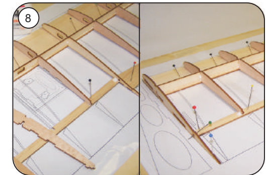
8 Rippen F 11 bis F 16 einleimen, Beplankungsteile dabei auf dem Baubrett aufnadeln
