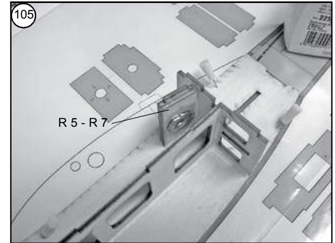
Bild 105 - Vorbereitete Flächenhalterung R 5 - R 7 einkleben.
