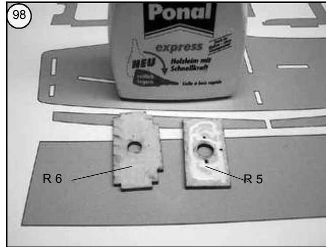
Bild 98 - Die Aufdupplung R 5 auf die Flächenhalterung R 6 kleben.
