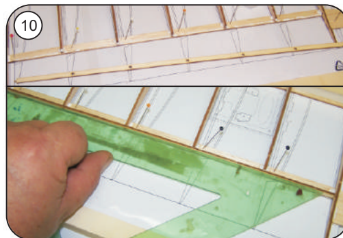
10 Querruder- Anschlag F 18 einkleben und gerade ausrichten
