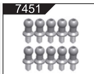
7451 Kugelköpfe M3-4.9x10.6 (10)
