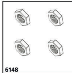
6148 Radmuttern 17mm (4)
