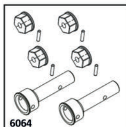
6064 Radachsen/ Felgenmitn.
