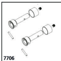
7706 Radachsen/ Felgenmitn.
